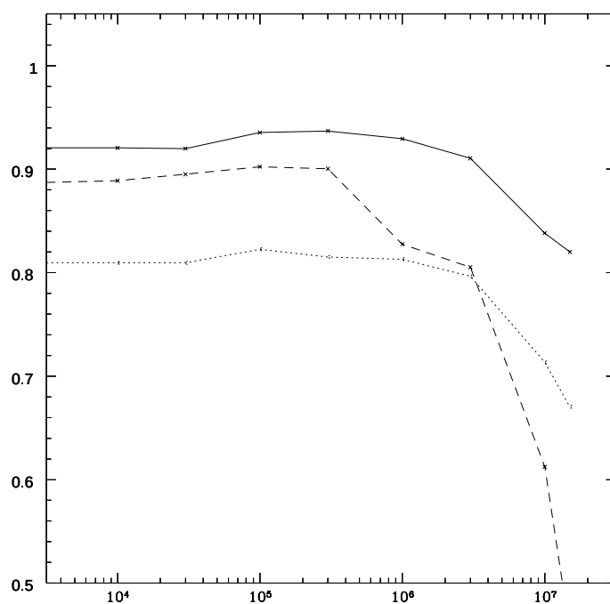
図 3: J270 FET バッファのゲイン・周波数関係。実線が J270 で V_{SS} = 15.0V の時、点線が V_{SS} = 5.0V のとき。破線が J230 で V_{DD} = 15.0V のとき。
