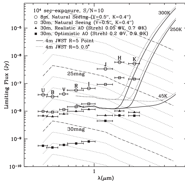
図 3: 地上 30m/4m 宇宙望遠鏡の比較。黒丸は AO なしの地上 8 メートル望遠鏡、緑四角は口径 30 メートルの時。青三角は、地上 30 メートルで現在の技術レベルの AO を使ったとき (Strehl 比 0.7 @ K , 0.05 @ V )。紫四角は理想的な AO が実現したとき (Strehl 比 0.9 @ K , 0.2 @ V )。実線は点源に対する 4m 宇宙望遠鏡の感度。波線は 0.5'' に広がった天体に対する感度。望遠鏡の温度が 45K, 250K, 300K の時の限界等級をそれぞれ緑、赤、水色で示した。
