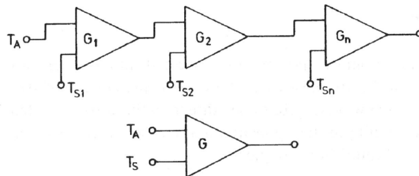
図 5.3 カスケード増幅器。
