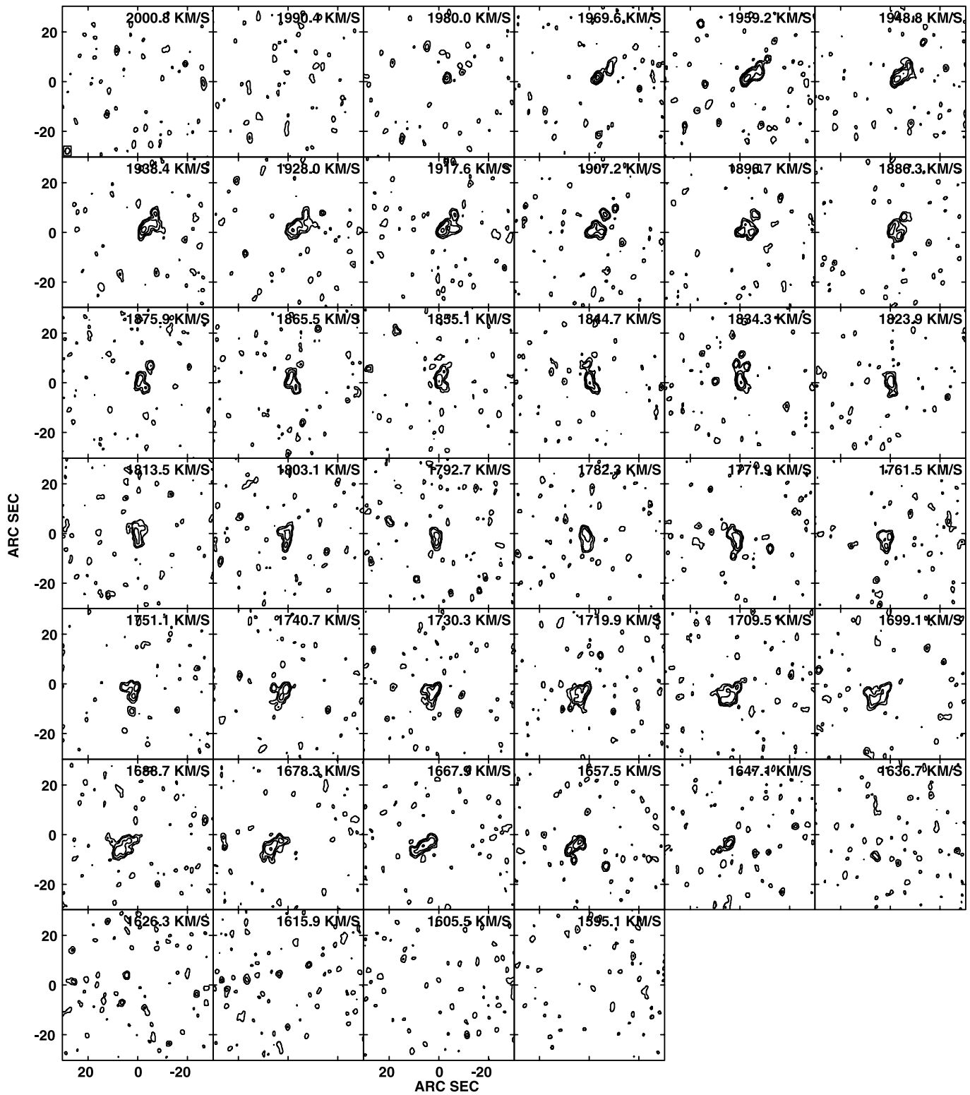
Fig. A1. (Continued.) NGC 4536: Lowest \sigma = 0.5 K.
