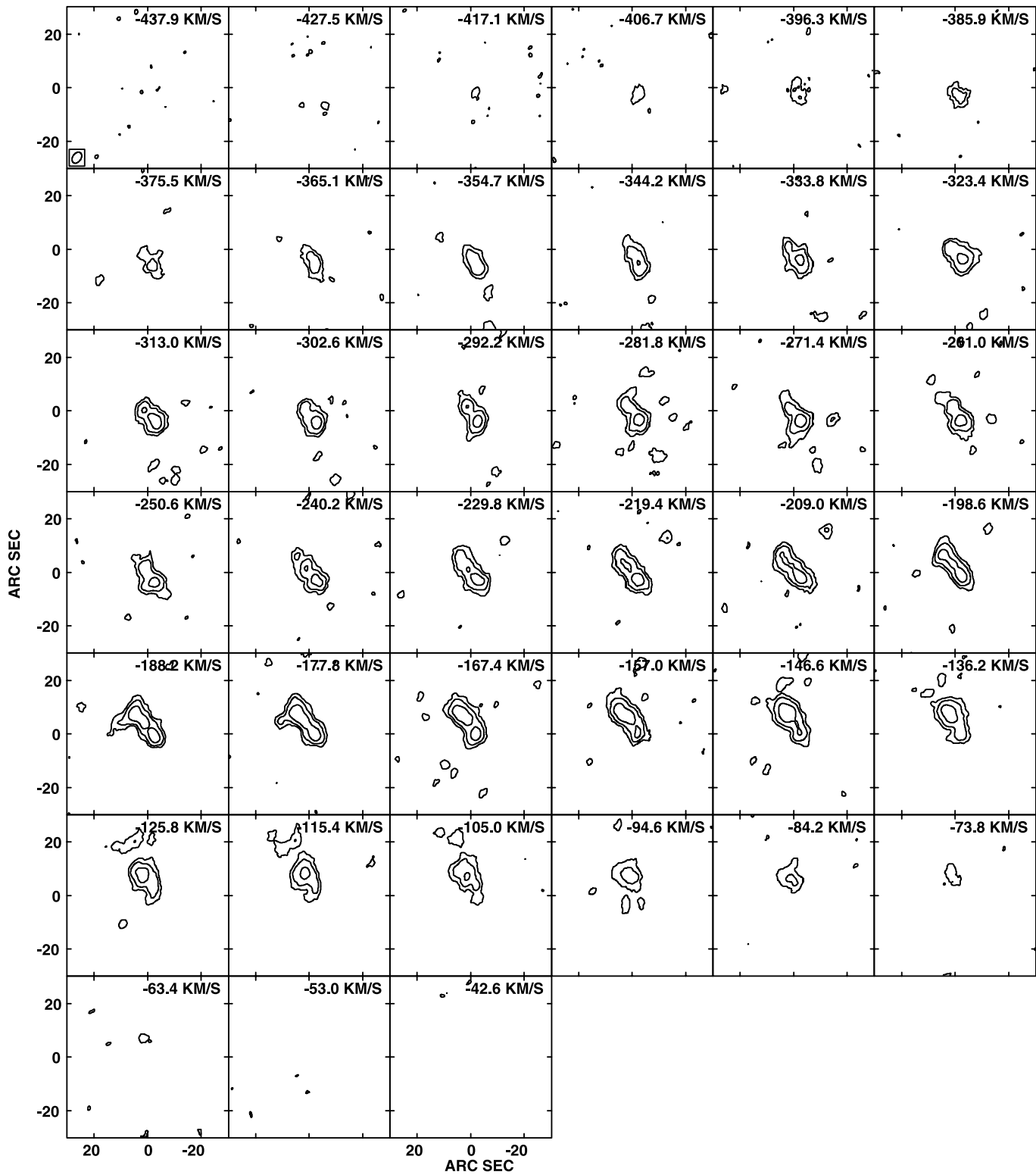
Fig. A1. (Continued.) NGC 4569: Lowest \sigma_l = 0.5 K.
