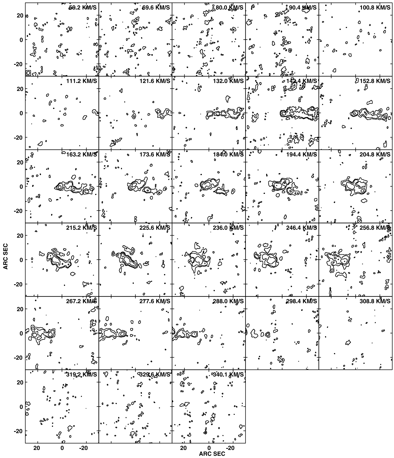
Fig. A1. (Continued.) NGC 4402: Lowest \sigma = 0.5 K.
