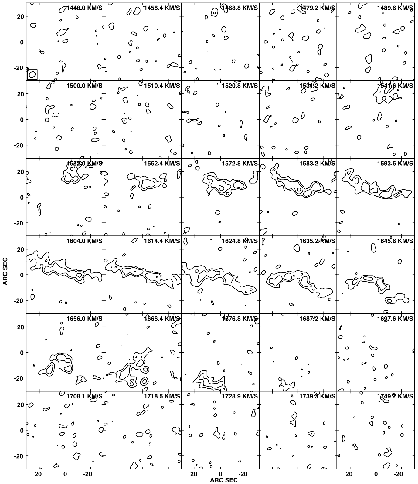
Fig. A1. (Continued.) NGC 4689: Lowest cl = 0.125 K.
