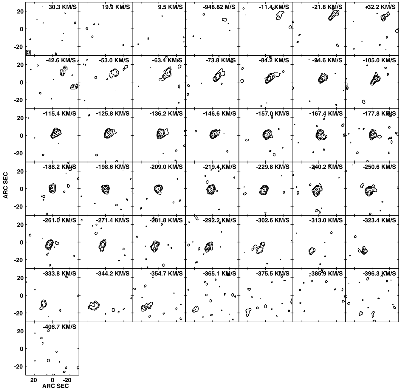
Fig. A1. (Continued.) NGC 4419: Lowest cl = 0.5 K.
