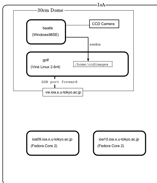
図 1: 計算機群の構成
